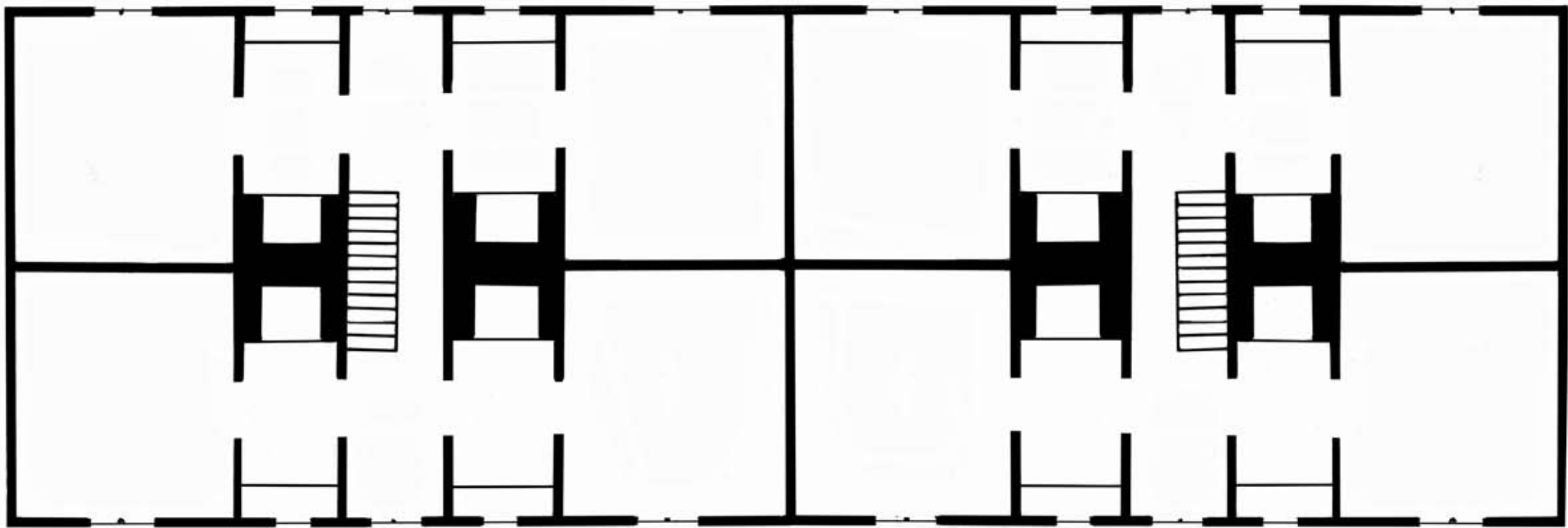
Johan Ohlsens gate 8, Militærhospitalet, Stavern - rekonstruksjon av grunnplan 2. etasje
